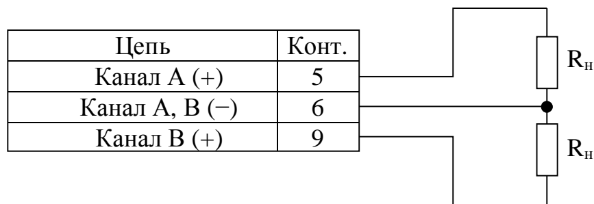
Рисунок 2.5 – Схема подключения внешней нагрузки R_n к контактам разъема « ТОКОВЫЙ ВЫХОД »
