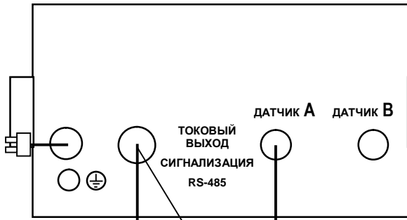
Блок преобразовательный щитового исполнения (вид сзади)
